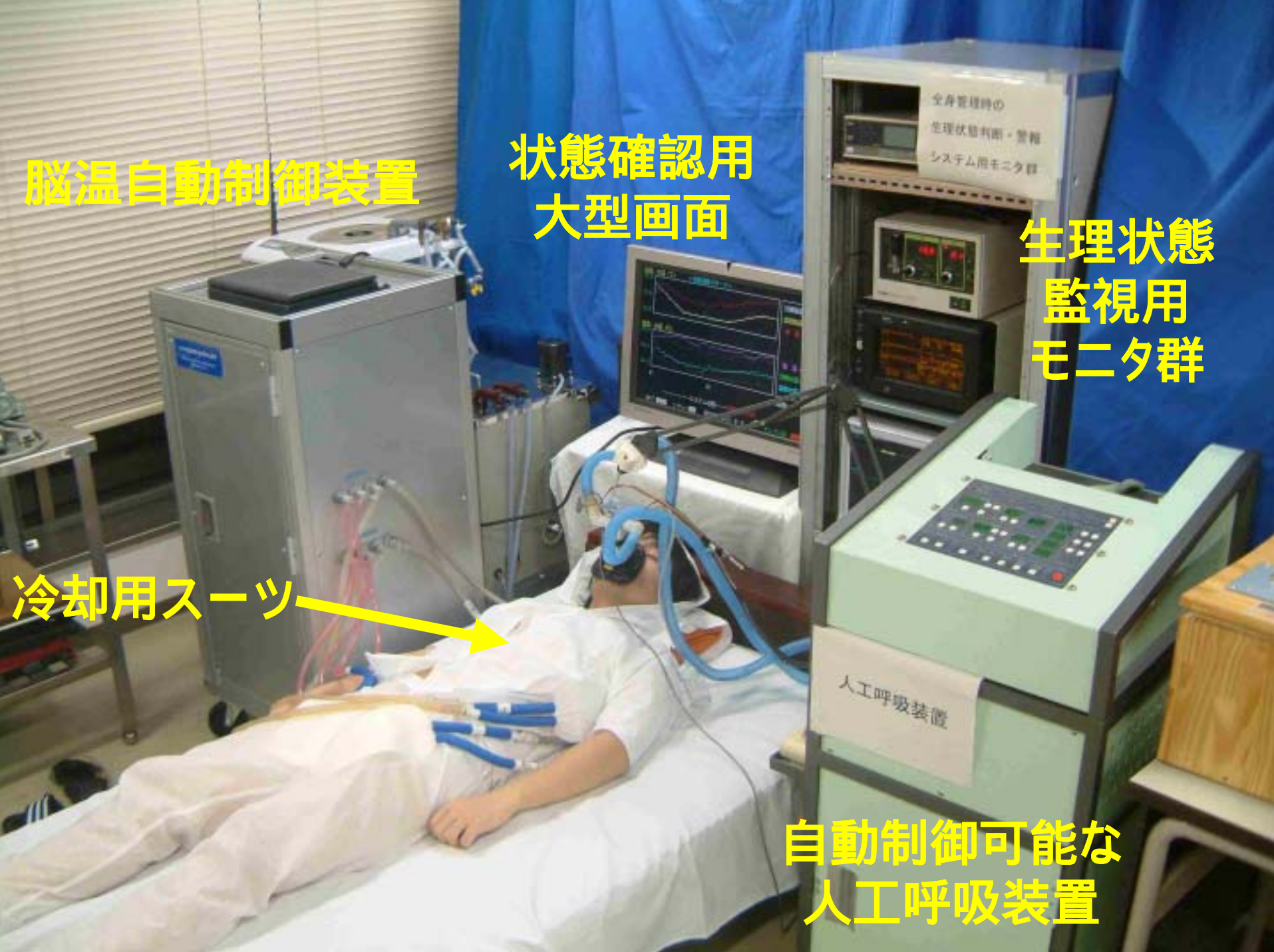
図2 脳低温療法時の脳温・呼吸自動制御システム
