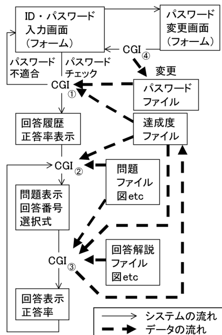
図 1 Web-Learning システムの流れ図
